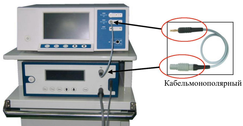
а) Оборудование DS.Surg.Argon и DS.Surg Plus
