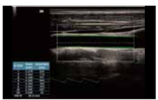
R-VQS
