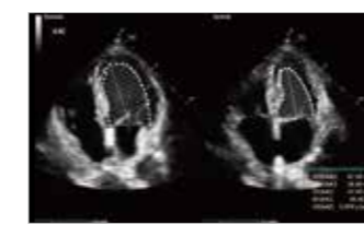
AutoEF
